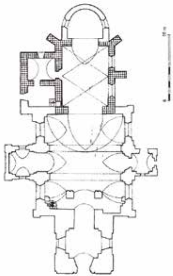
Rzut kościoła św. Jana w Koźminku. Źródło: J. Tomala, Murowana architektura romańska i gotycka w Wielkopolsce, t. I Architektura sakralna, Kalisz 2007
